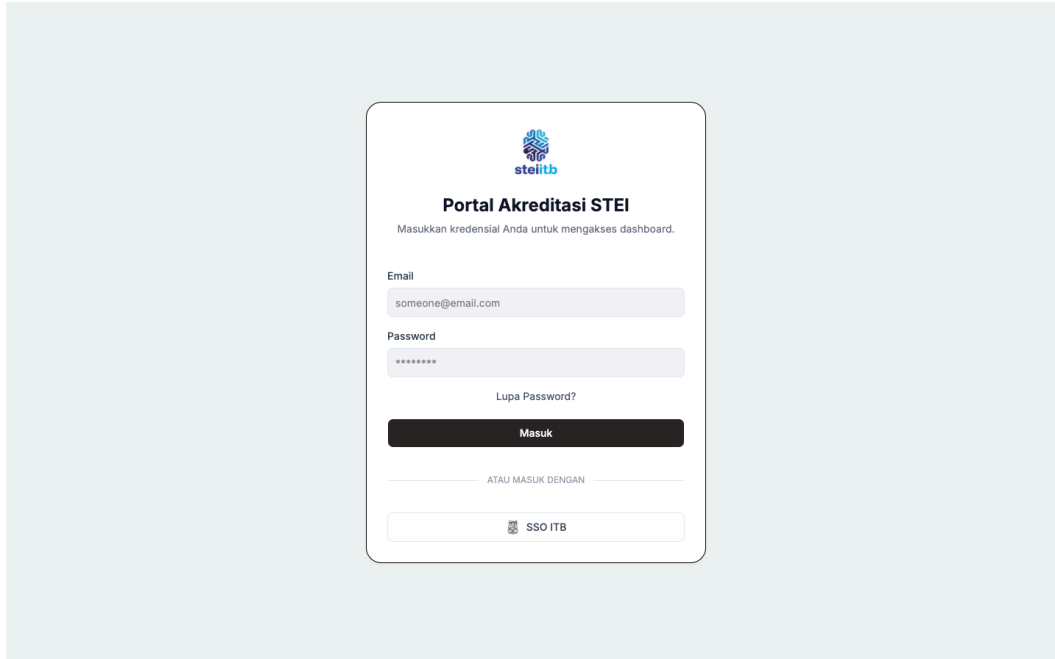
Gambar 8.1 Page Login
